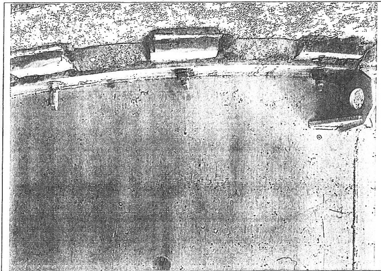
Hianyó lehorgonyzó csavar az ajtó alatt
