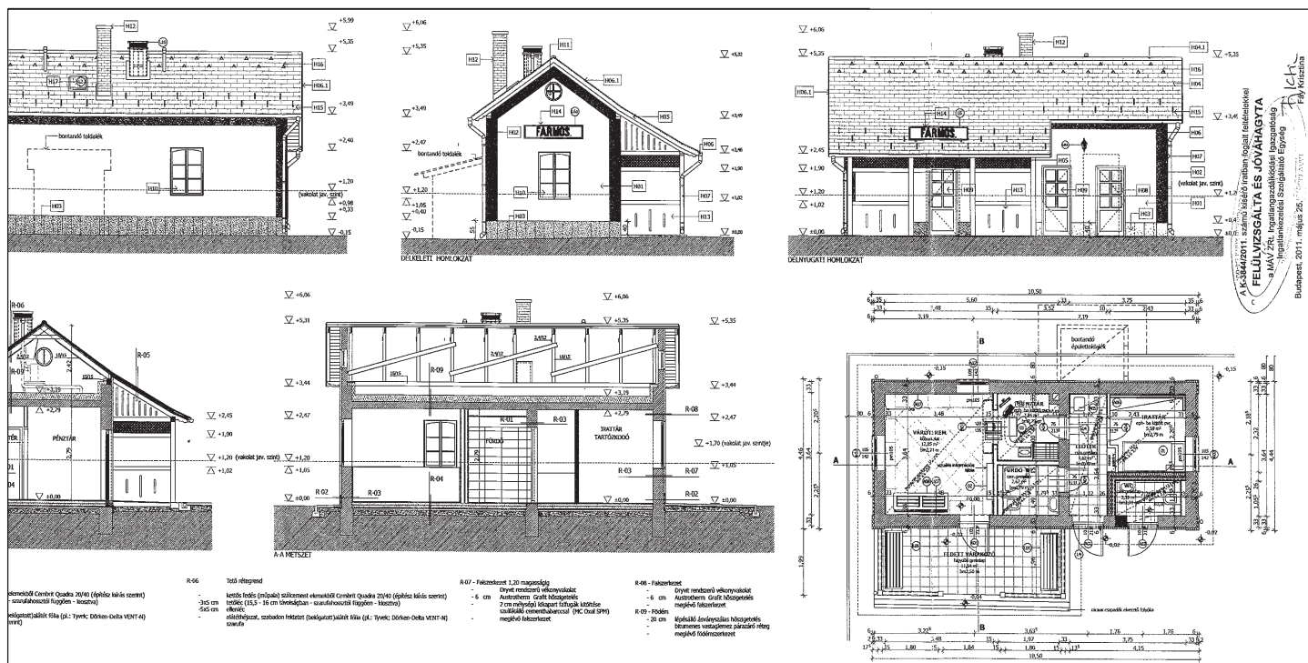
A farmosi vasútállomás tervrajzának részlete.
