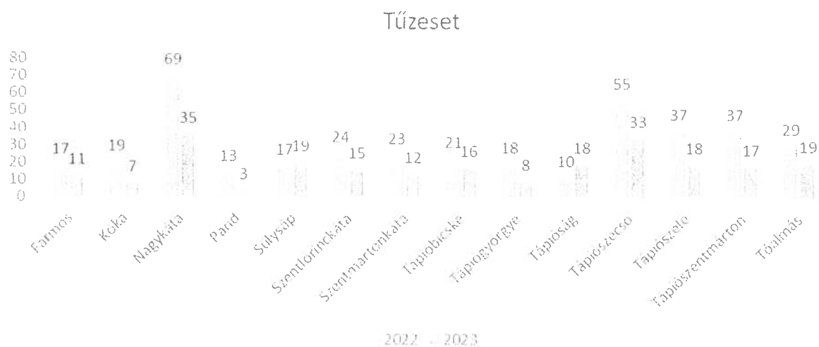
3.sz. ábra 2022 – 2023 tűzesetek alakulása
